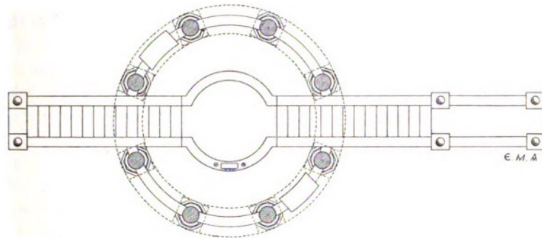
Σχ. 242. Ἀποκατάταξις τοῦ διαγράμματος τοῦ δευτέρου τῆς Ἁγίας Σοφίας Ἄμβωνος. Κλίμαξ=1½.
